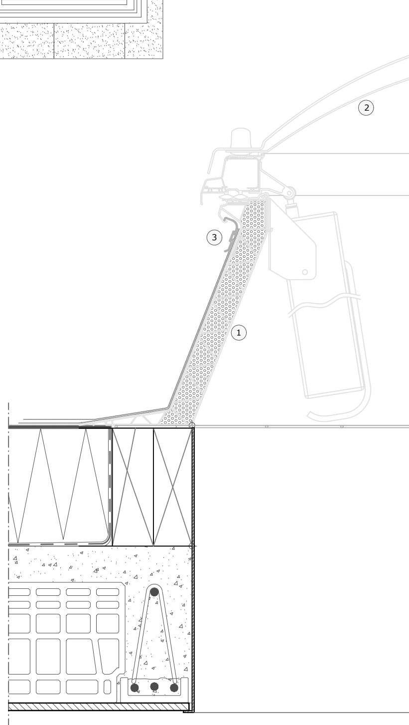
Section A-A 1:5
