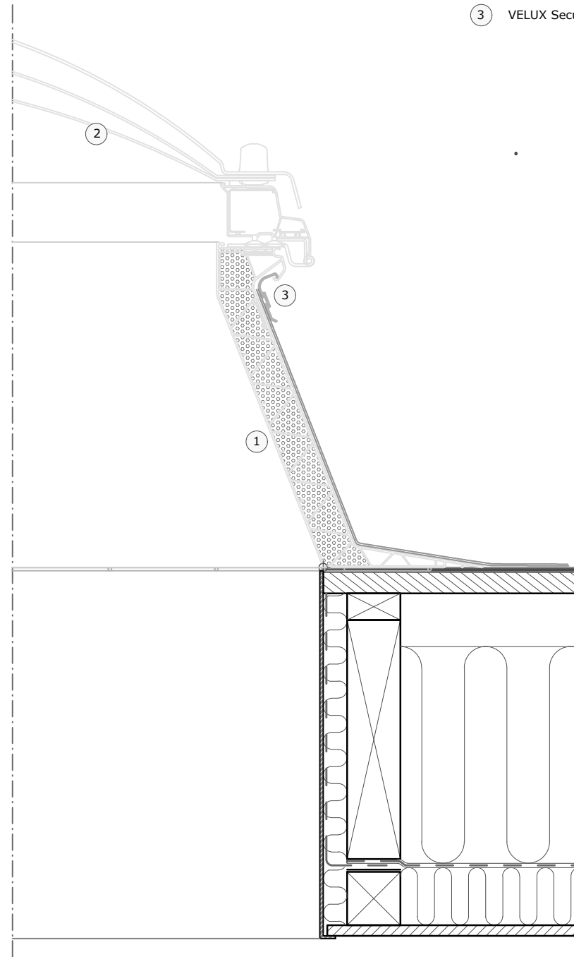
Section A-A 1:5
